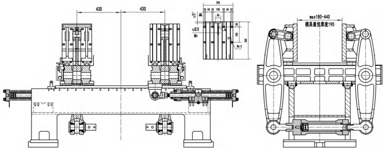
HS II -2L (挤出中空吹塑设备)
