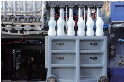
HT-六模头 HT-Triple Die Head
