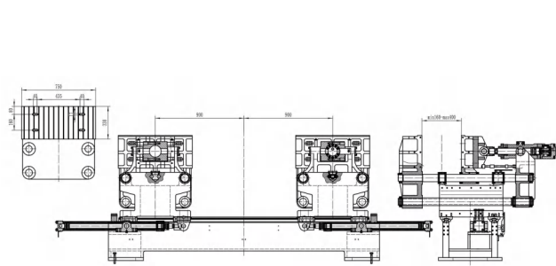
HTS II -8L（挤出中空吹塑设备）
