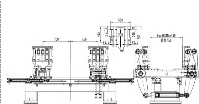
HS II -20L（挤出中空吹塑设备）
